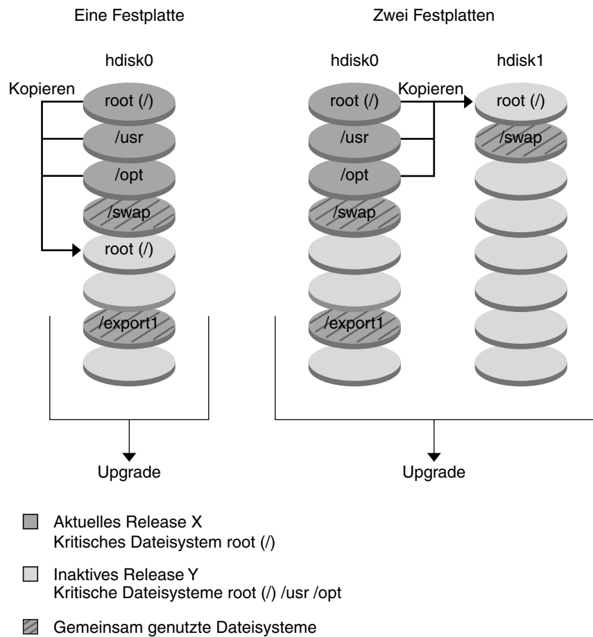
ABBILDUNG 30-3 Erstellen einer inaktiven Boot-Umgebung — Zusammenführen von Dateisystemen
