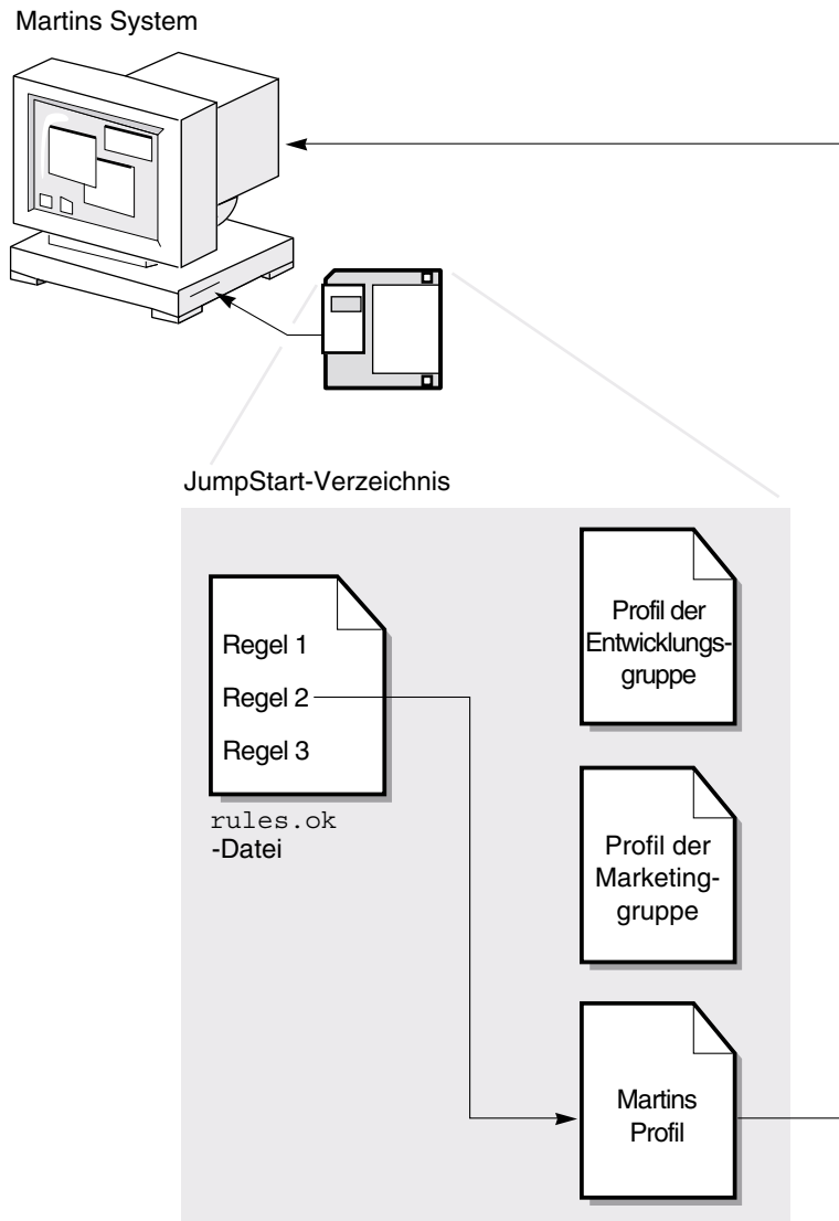
ABBILDUNG 22-1 So läuft eine JumpStart-Installation ab: Beispiel für nicht vernetzte Systeme
