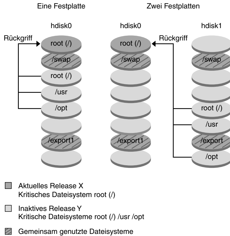
ABBILDUNG 30–7 Zurückgreifen auf die ursprüngliche Boot-Umgebung
