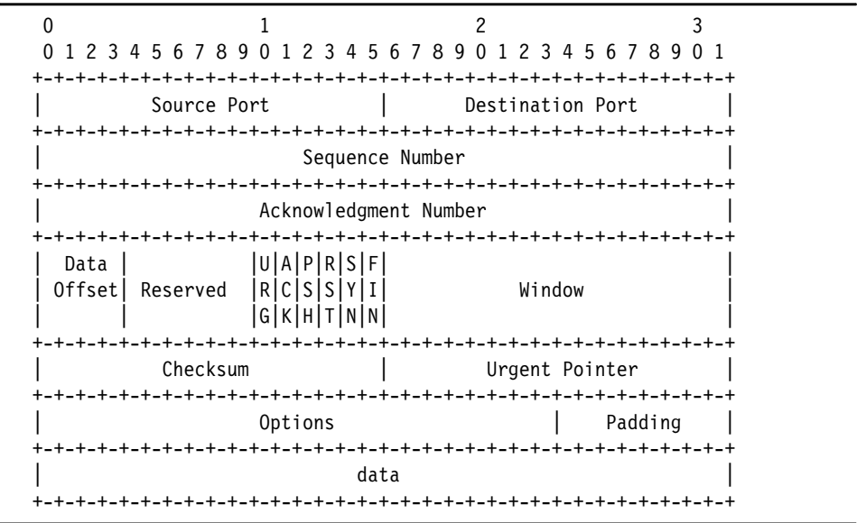
Example 2-3 TCP header
